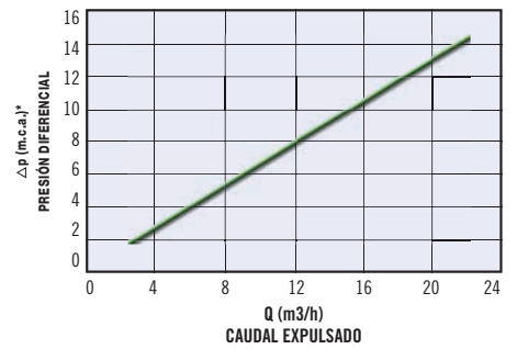
Función desgasificación
