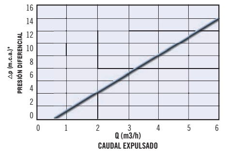
Función desgasificación
